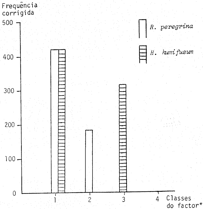
Fig. 2 — Perfis das frequências corrigidas de Rubia peregrina e Hypericum humifusum para o factor «Frequência dos tratamentos herbicidas»
