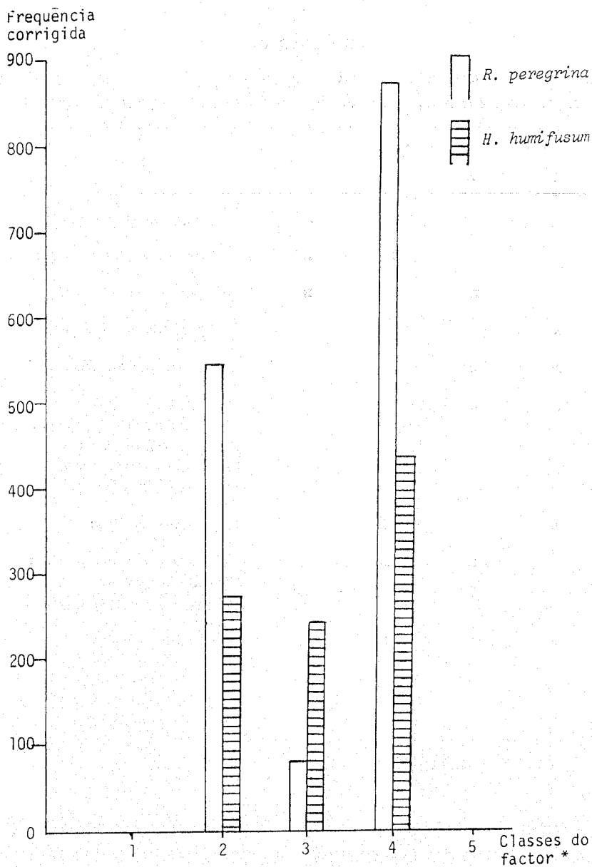
Fig. 1 — Perfis de frequências corrigidas de Rubia peregrina e Hypericum humifusum para o factor «Sistema de controlo das infestantes».
